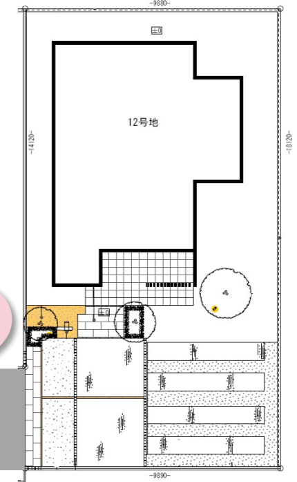
敷地配置図
